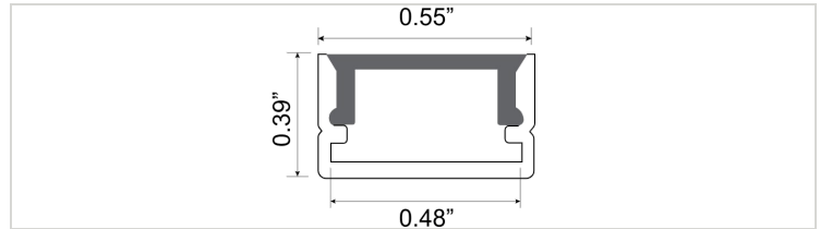
FIG. 02 · CROSS-SECTION
