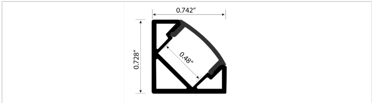
FIG. 02 · CROSS-SECTION
