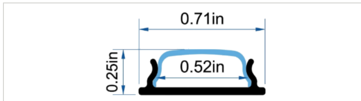
FIG. 02 · CROSS-SECTION
