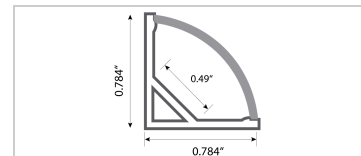
CURVE45 DLDT-S-CRV45
